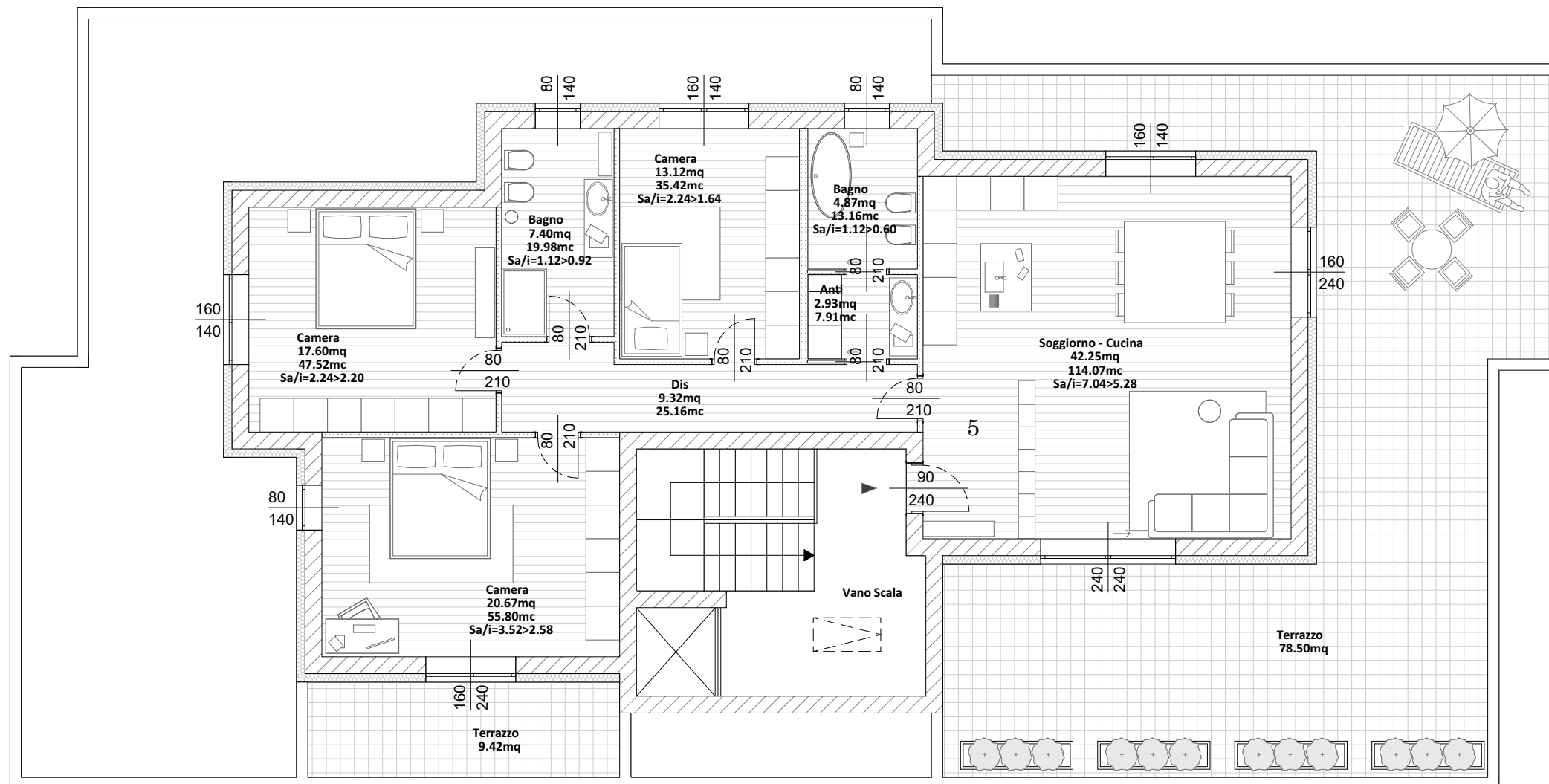
PIANTA PIANO SECONDO Sc.1:100
